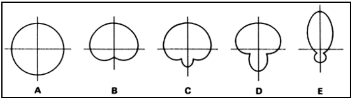
Figura 6. Patrones polares de los diferentes tipos de micrófonos, los cuales son como sigue: A) omnidireccional, B) cardioide, C) hipercardioide, D) supercardioide y E) shotgun. Tomado de WICKSTROM (1982), reimpresso con permiso de Elsevier.
